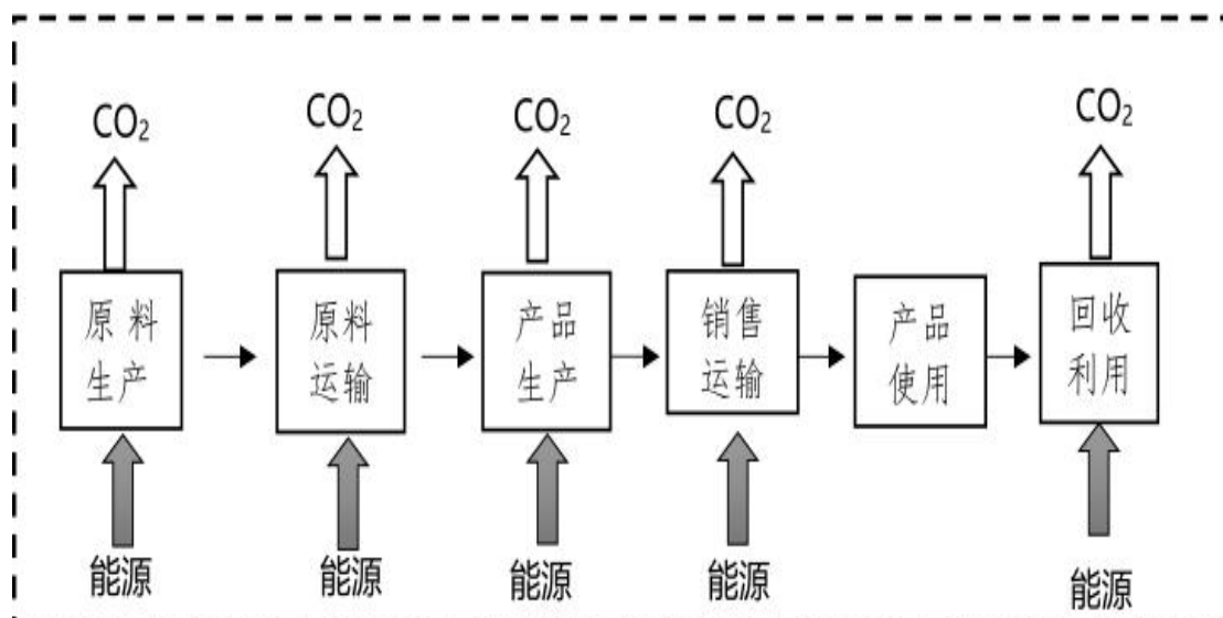
图 2 滚动轴承产品生命周期评价边界图
